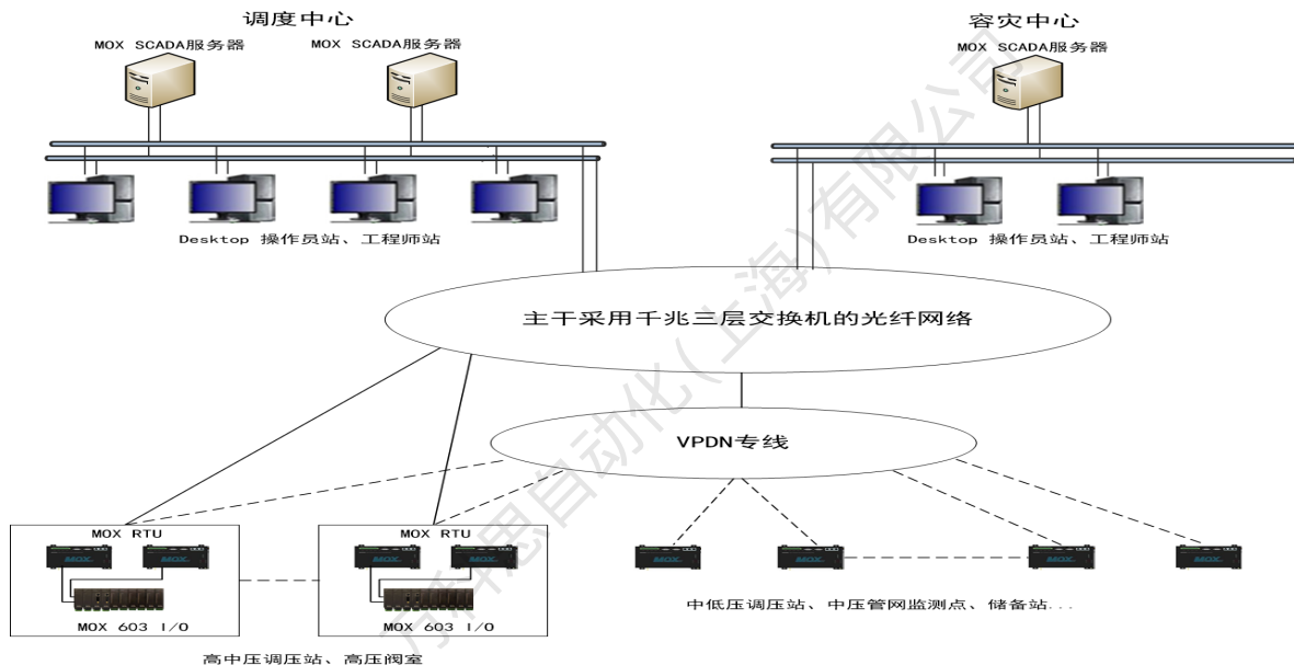
城市燃气SCADA系统架构图
